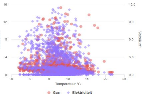
Elektriciteitsverbruik per dag en per uur
